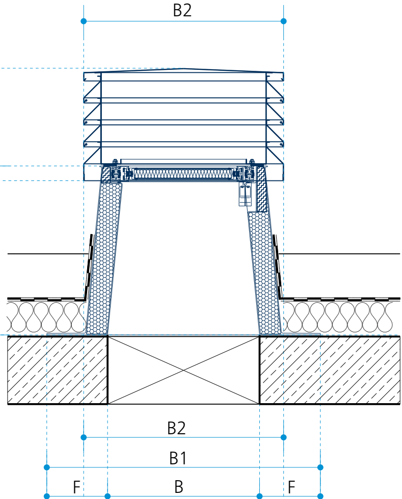
Schnitt A-A
